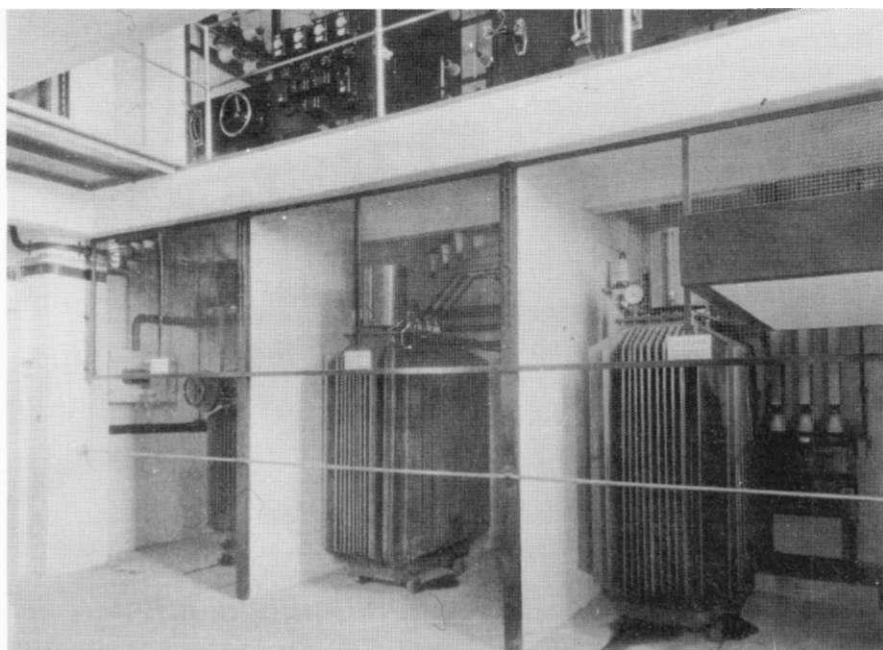
Krafttransformatorer i undre våningen av ställverket. Längst t.v. spänningsregulatorn
